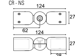
B-173 €► BX.336 • Raccordo regolabile per tubo Ø 19 mm. • Adjustable connector for Ø 19 mm tube. • Verbinder für 19 mm Rohr Verstellbar. CR - NS
