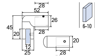
B-165 €► BX.334 • Raccordo a 90° per tubo Ø19 mm. • 90° connector for 19 mm tube. • Rohrverbinder 90° für Rohr Ø 19 mm. CR - NS
