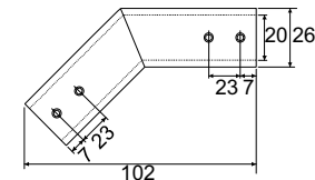
B-184 €► BX.335 • Terminale a muro 45° per barre fermavetro Ø 19 mm. • Wall fixing bar 45° end for Ø 19 mm tube. • Drehbar Halterungen 45° für Stabilisationsstange. CR - NS
