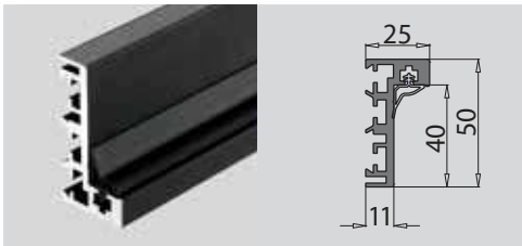
P-030/P-031 Door jamb / Zarge - Jamba de puerta - Encadrement
