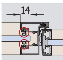
B-146 Glass gaskets mm 8/10 mm Glasdichtungen mm 8/10 mm Guarnición mm 8/10 Joint pour verre de 8/10 mm
